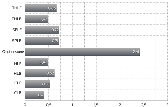
Resistencia a la Flexión (N/mm²)
