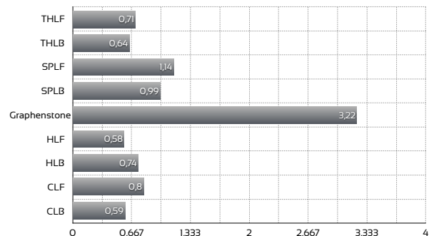
Resistencia a Compresión (N/mm²)
