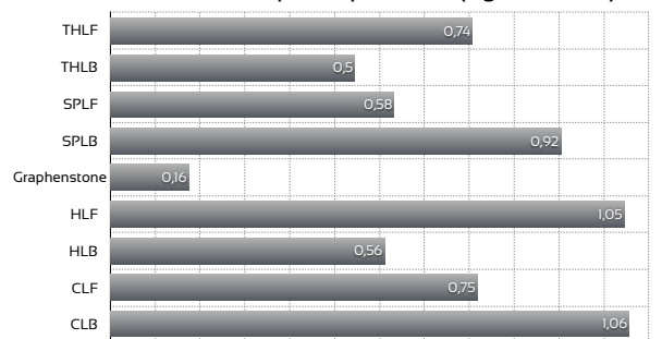
Absorción por capilaridad (kg/m² min 0,5 )
