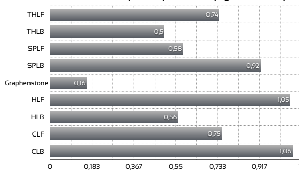
Absorción por capilaridad (kg/m 2 min 0,5 )
