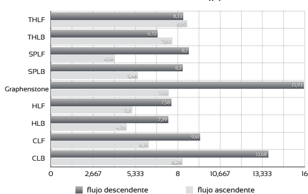
Permeabilidad (μ)
